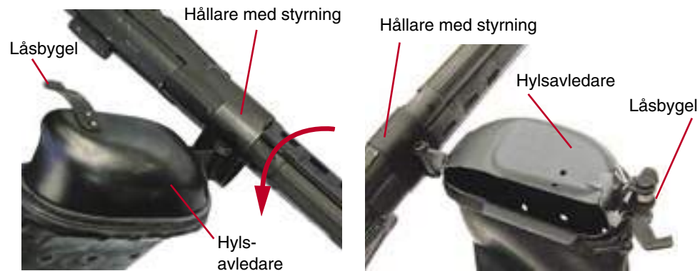
Fastsättning av hylsfångare Ak 4 Ak 4 B
