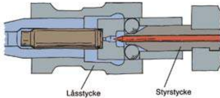
(4) Mekanismens bakåtgående rörelse
