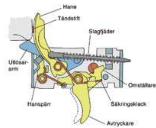
(3) Patronvis eld – Avfiring
