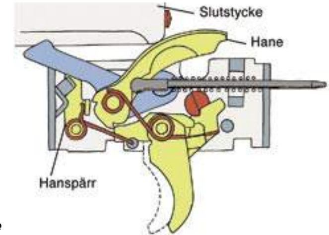
(5) Patronvis eld – Återgående rörelse
