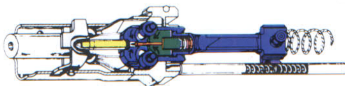
Rohr und Verschuß entriegeln
