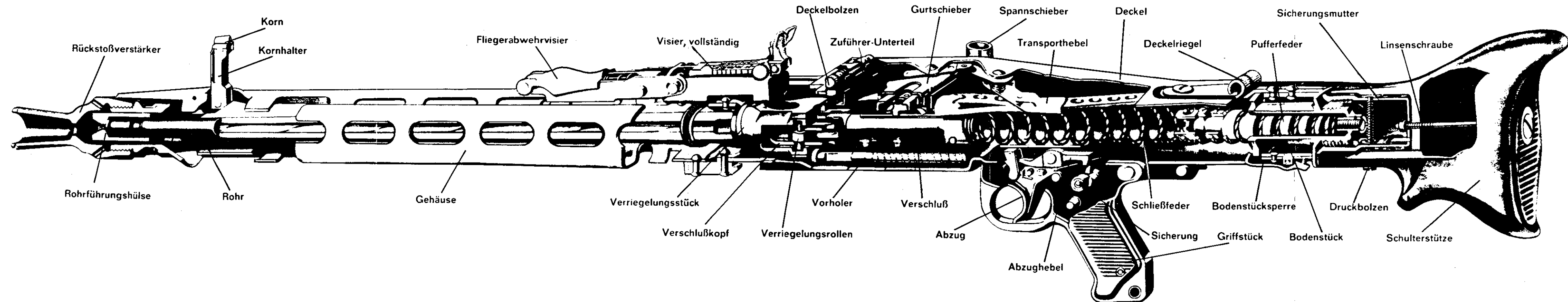
Schnittbild
