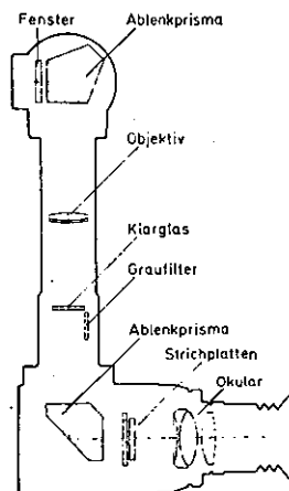
ZF-MG, optischer Aufbau
