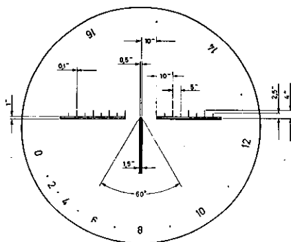
Zeichnungsmaße zum Strichbild
