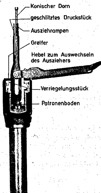
Ausziehen einer steckengebliebenen Patrone oder Patronenhülse
