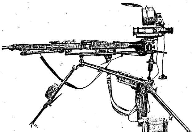
Infrarot-Zielgerät auf Feldlafette-MG
