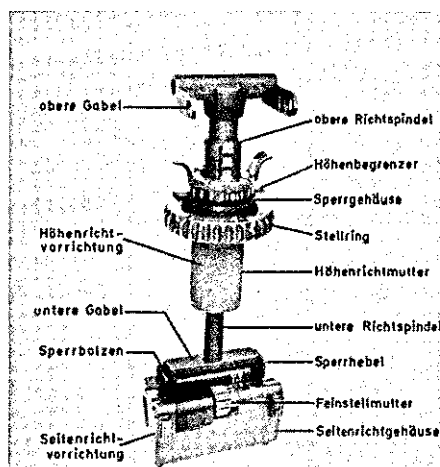
Richtvorrichtung
