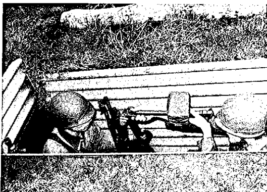
Vorderstütze ausschwenken (im Kampfstand)
