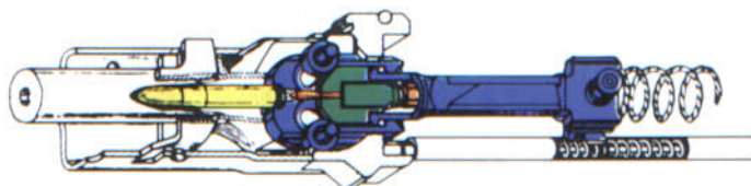
Rohr mit Verschluss verriegelt
