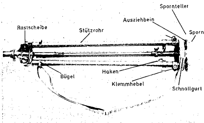
Stützbeine und Tragevorrichtung
