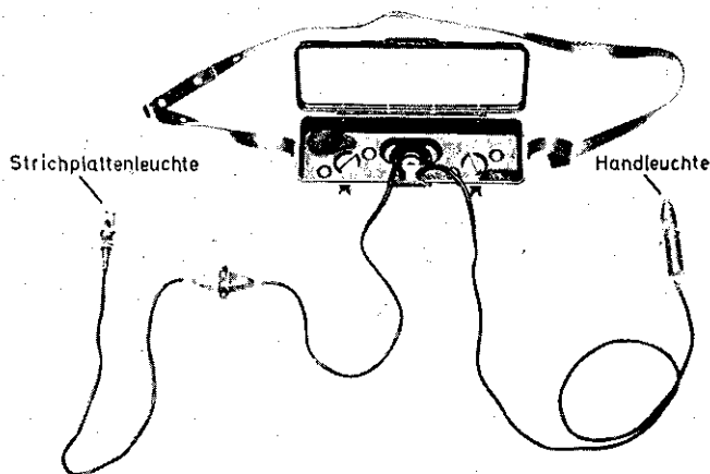
Beleuchtungseinrichtung
