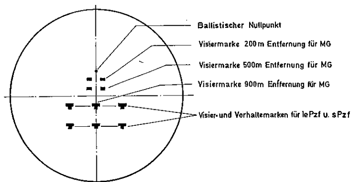
Strichbild des Bildverstärker-Zielfernrohrs
