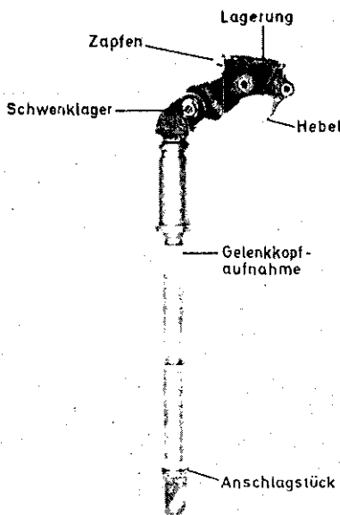
Gelenkkopf mit Gelenkkopfaufnahme
