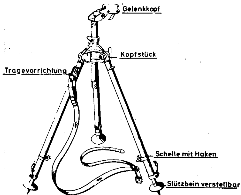
Fliegerdreibein
