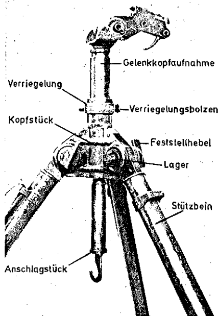
Kopfstück mit Stützbeinen
