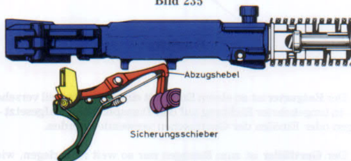
Abzugshebel hält Verschuß in hinterer Stellung
