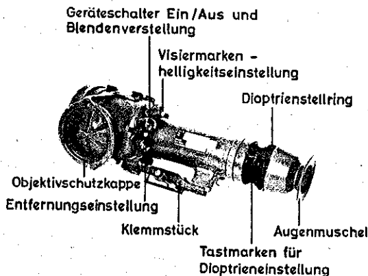
Bildverstärker-Zielfernrohr, linke Seite
