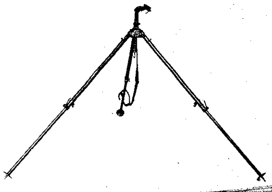
Großer Aufstellwinkel der Stützbeine (Fliegerdreibein in standsicherster Stellung)
