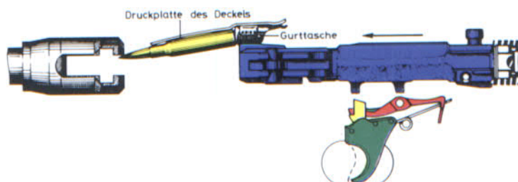
Ausstoßen der Patrone aus dem Gurt
