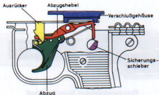
Stellung des Sicherungsschiebers auf „F“
