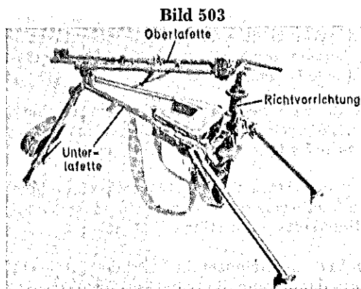
Feldlafette-MG
