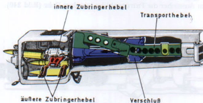
Transporthebel bei beginnendem Verschlußvorlauf
