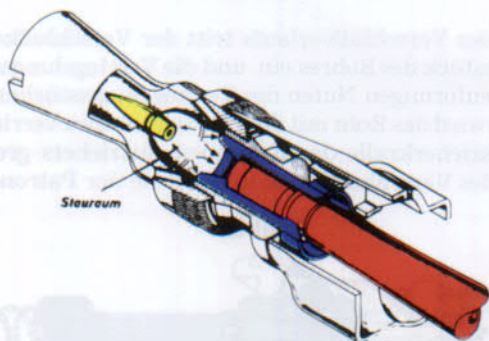
Rückstoßverstärkung
