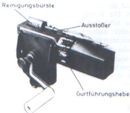
Entgurten
