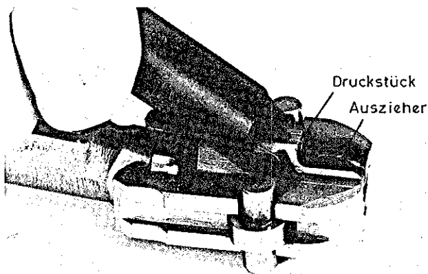
Auswechseln des Ausziehers
