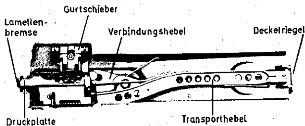
Deckel mit Transporthebel, Verbindungshebel und Gurtschieber
