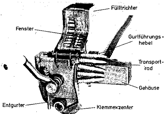
Gurtfüller
