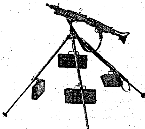
Maschinengewehr auf Fliegerdreibein
