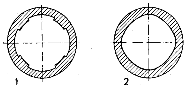
Rohr mit Zügen und Feldern (1) und Polygonrohr (2)
