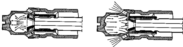
Wirkungsweise des Manöverpatronengeräts
