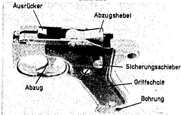
Griffstück
