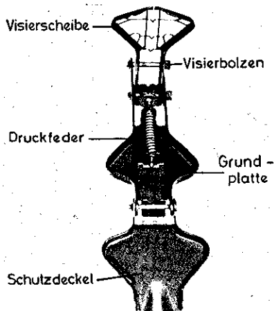
Fliegerabwehrvisier, von vorn oben gesehen
