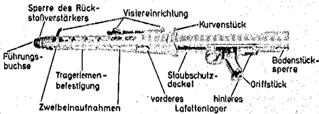
Gehäuse
