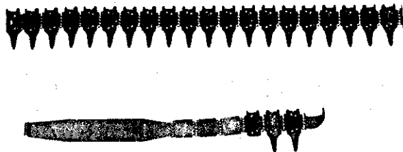
Teilansicht des Patronengurts DM1 und Einführstück (leer von unten gesehen)
