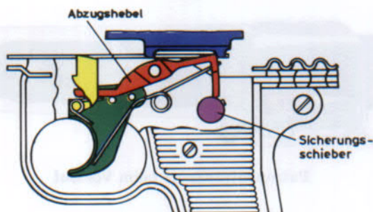
Stellung des Sicherungsschiebers auf „S“
