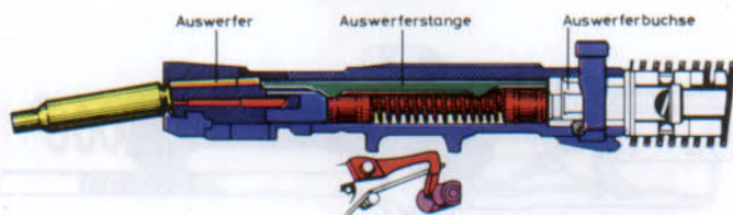
Auswerfen der Patronenhülse
