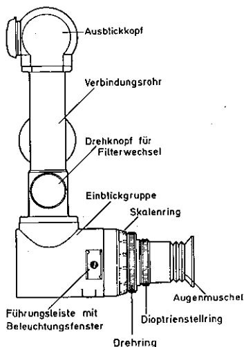
ZF-MG, mechanischer Aufbau
