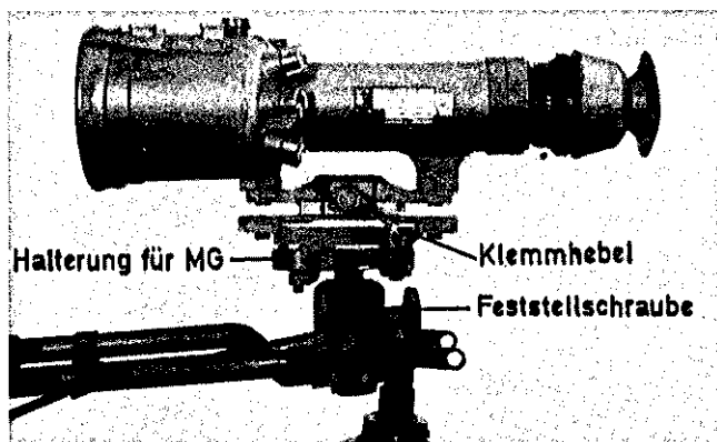
Bildverstärker-Zielfernrohr auf Feldlafette-MG Klemmhebel nach unten gedrückt
