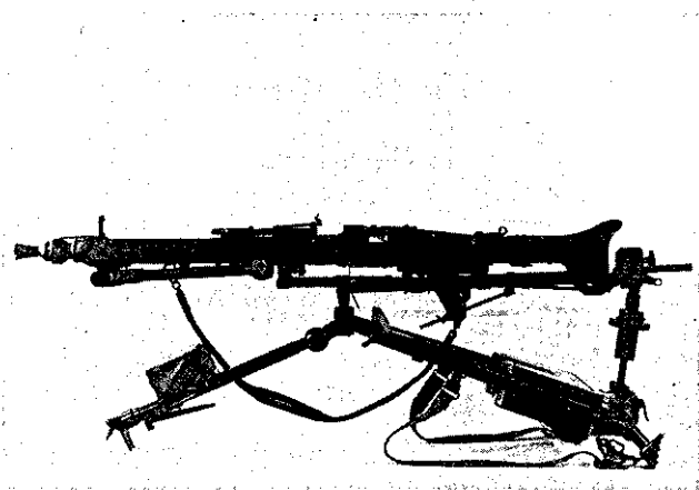
MG auf Feldlafette mit eingeklappten Hinterstützen
