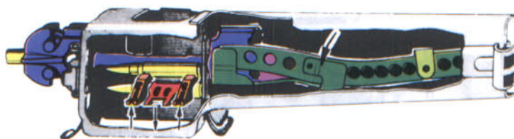
Patronentransport beim Vorlauf
