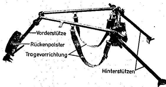
Unterlafette (Stützen ausgeklappt)
