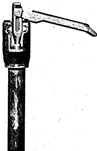
Ausziehen einer Patronenhülse (Hülsenboden abgerissen)
