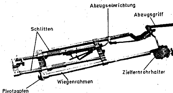
Oberlafette mit Wiegenrahmen, Schlitten und Abzugseinrichtung
