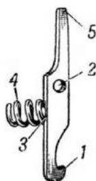
Рис. 18. Защелка спусковой скобы: 1 — зуб; 2 — отверстие для оси; 3 — гнездо; 4 — пружина защелки; 5 — верхний конец защелки
