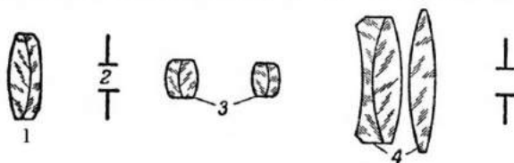
Рис. 96. Оптическая схема прицела: 1 — двухлинзовый объектив; 2 — диафрагма с перекрестьем; 3 — оборачивающая система; 4 — трехлинзовый окуляр
