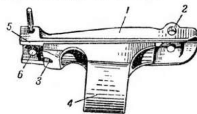
Рис. 11. Колодка прицела:
