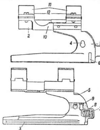
Рис. 102. Общий вид кронштейна:
