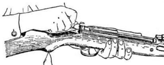
Рис. 62. Отделение ударно-спускового механизма
