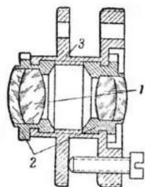
Рис. 99. Разрез оборачивающей системы:
