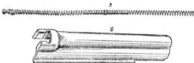
Рис. 22. Запирающий механизм:
