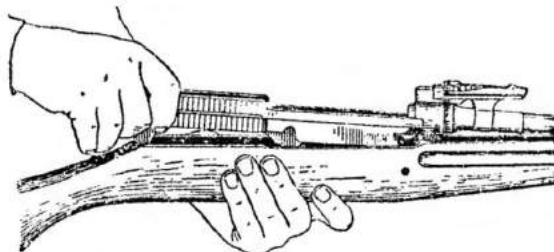
Рис. 67. Отделение ложи от ствола
