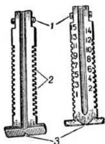
Рис. 12. Прицельная планка:
