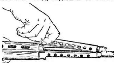
Рис. 64. Отделение верхнего кожуха
