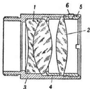
Рис. 101. Разрез окуляра прицела:
