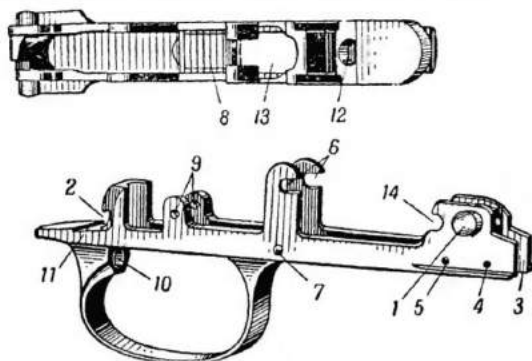
Рис. 30. Спусковая скоба:
