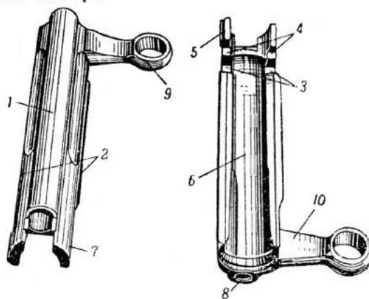
Рис. 26. Стебель затвора: 1 — гребень; 2 — направляющие выступы; 3 — нижние вырезы; 4 — срезы; 5 — выступ; 6 — жолоб; 7 — задний вырез; 8 — гнездо; 9 — рукоятка; 10 — номер.
