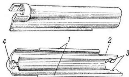
Рис. 28. Крышка ствольной коробки:
