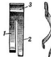
Рис. 37. Пружина спусковой тяги: 1 — изогнутое короткое перо; 2 — длинное перо; 3 — выгнутый конец
