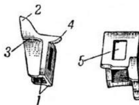
Рис. 19. Отражатель: 1 — боковые выступы; 2 — верхний выступ; 3 — ограничительный выступ; 4 — задний выступ; 5 — паз.
