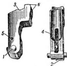
Рис. 31. Курок:
