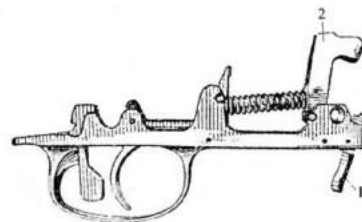
Рис. 87. Ударно-спусковой механизм:
