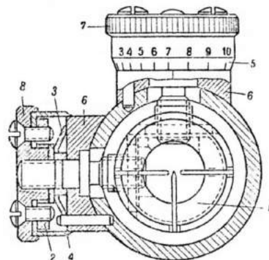
Рис. 100. Механизм установки углов прицеливания и боковых поправок:
