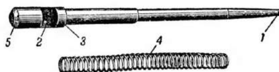
Рис. 25. Ударник с пружиной: 1 — боек; 2 — поперечный вырез; 3 — выступ; 4 — пружина; 5 — задний конец
