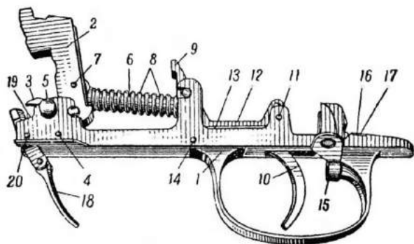
Рис. 29. Ударно-спусковой механизм:
