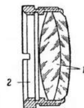
Рис. 97. Разрез объектива: 1 — линзы; 2 — оправа
