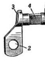
Рис. 38. Предохранитель: 1 — стержень; 2 — выступ головки; 3 — вырез для головки упора
