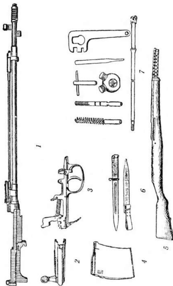
Рис. 2. Основные части самозарядной винтовки обр. 1940 г.: 1—ствол в собранном виде; 2—затвор; 3—ударно-спусковой механизм; 4—магазин; 5—ложа со ствольной накладкой; 6—штык; 7—приниждельность.
