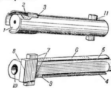
Рис. 23. Остов затвора:
